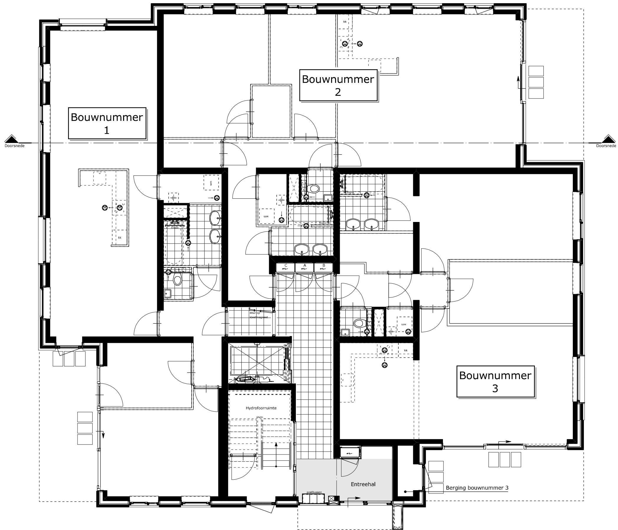
PLATTEGROND BEGANE GROND (peil=0)
