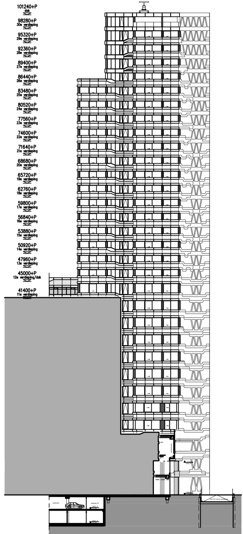
4. Zuid-Oost gevel
