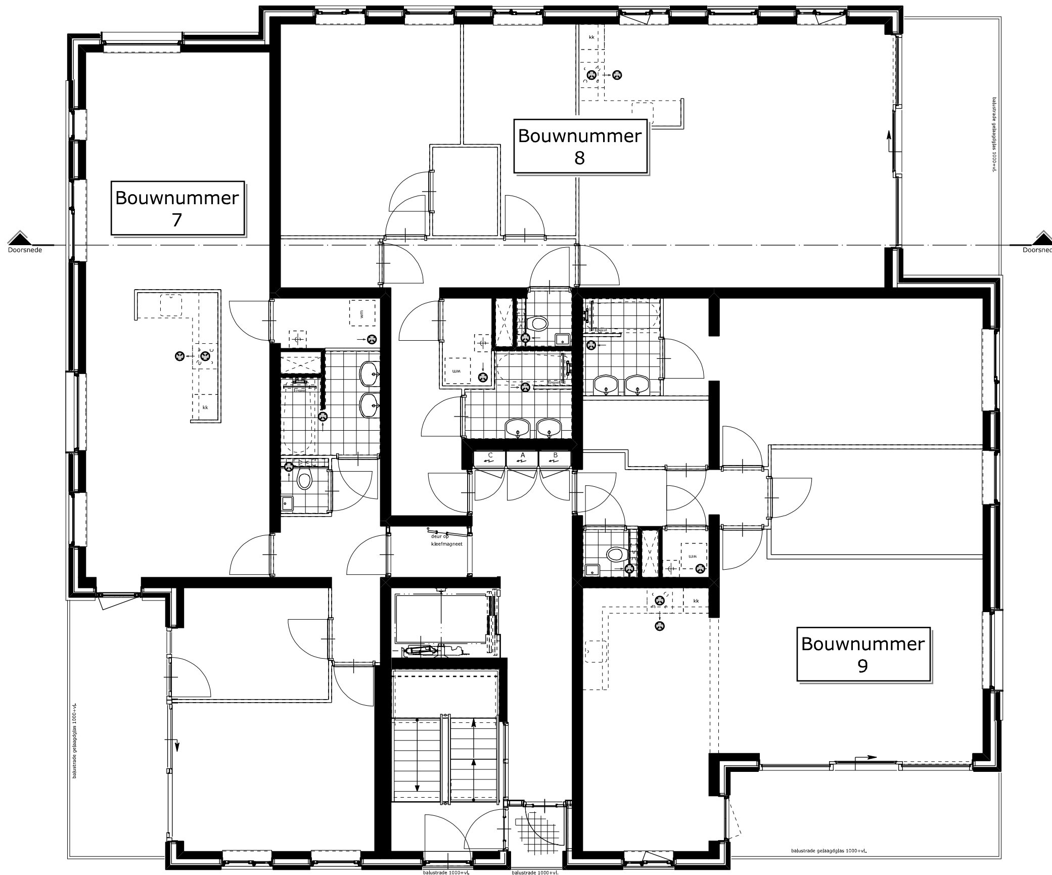
PLATTEGROND 2e VERDIEPING (5900+)
