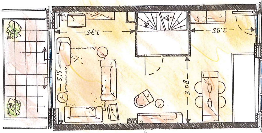
1 e verdieping
