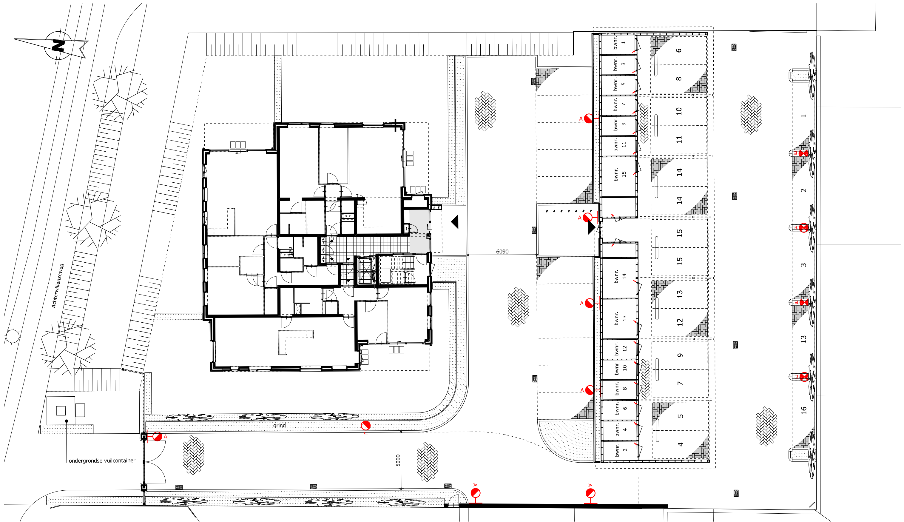
Situatietekening
