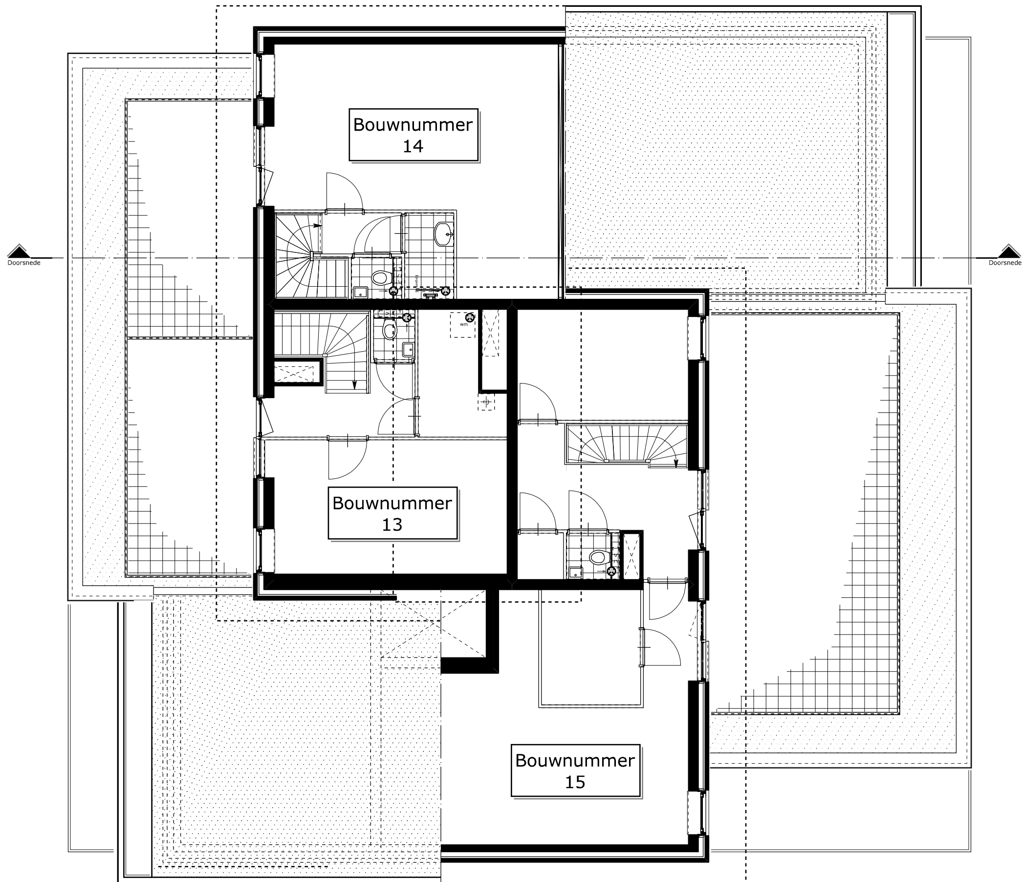
PLATTEGROND 5e VERDIEPING (14750+)
